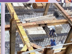
▲ 地樑模板組立完成
